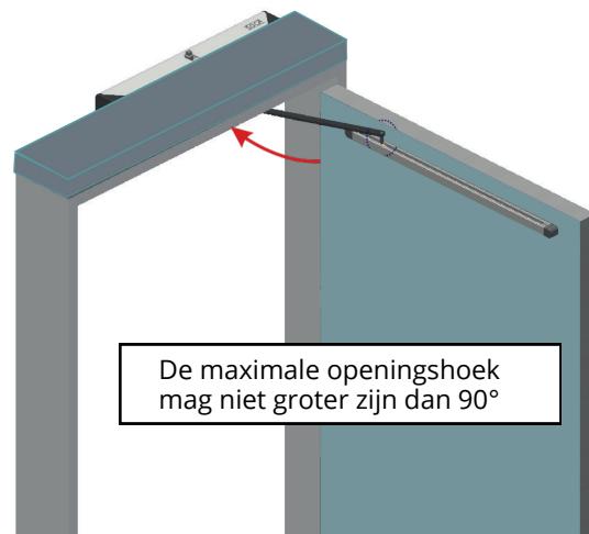
Installatie bij naar buitendraaiende deur
